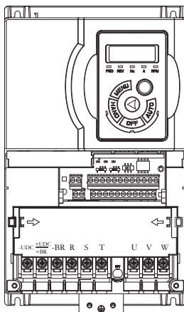
A0~A4 机箱主回路端子示意图
