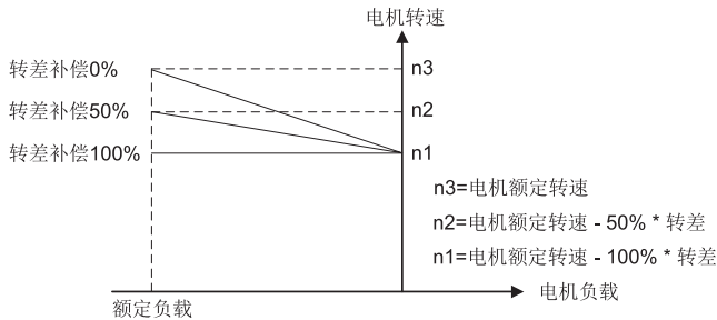
制动时的转差补偿
