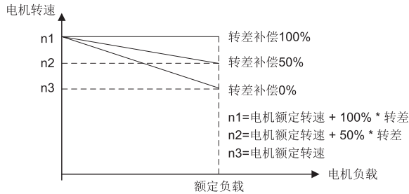
电动时的转差补偿
