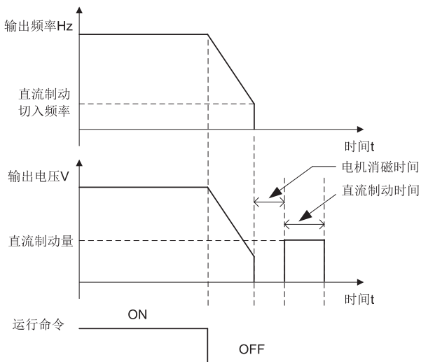
直流制动过程示意图:
