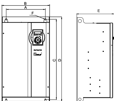
三相380V 30~90kW机型
