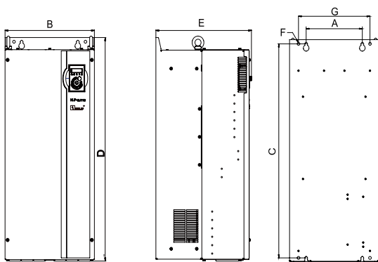
三相380V 110~160kW机型
