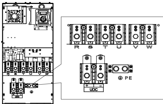
三相380V 110~160kW机型主回路端子示意图
