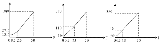
恒转矩曲线
