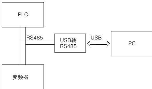
Modbus调试系统连线图
