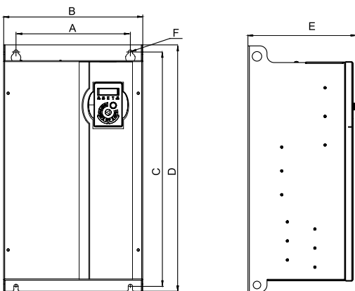
三相380V 30~75kW机型
