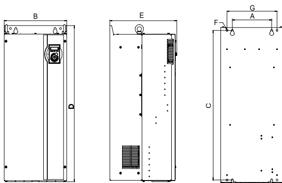
三相380V 90~220kW机型
