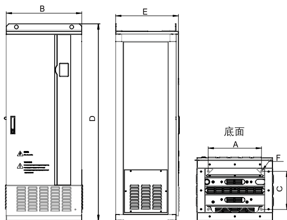
三相380V 250~415kW机型
