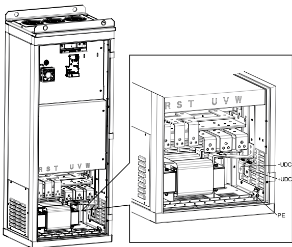
三相380V 250~415kW机型主回路端子示意图
