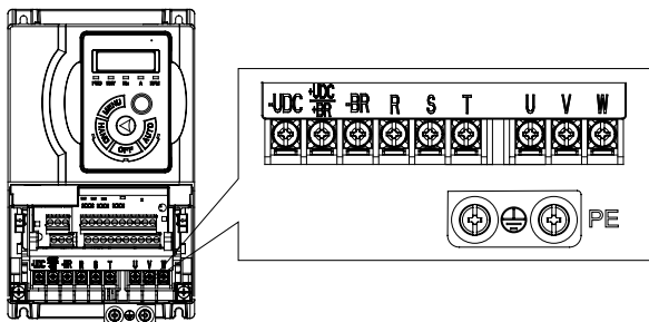
单\三相220V 0.37~3.7kW和三相380V 0.75~22kW机型主回路端子示意图
